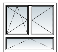
Dreh-Kipp / Dreh oder Dreh / Dreh-Kipp mit Unterlicht Kipp 2/3-1/3-Teilung Stulpausführung
