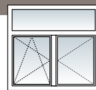
Dreh-Kipp / Dreh oder Dreh / Dreh-Kipp mit Oberlicht Fest 1/3-2/3-Teilung Stulpausführung
