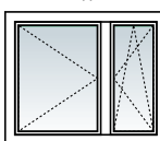
Dreh / Dreh-Kipp 2/3-1/3-Teilung Stulpausführung max. Flg.-Breite 1.240 mm
