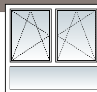
Dreh-Kipp/Dreh-Kipp mit Unterlicht Fest 2/3-1/3-Teilung
