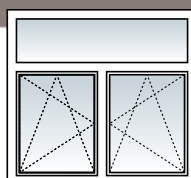
Dreh-Kipp/Dreh-Kipp mit Oberlicht Fest 1/3-2/3-Teilung
