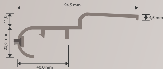
Abrollleiste
