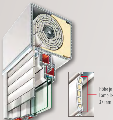
Aufsatzkasten
