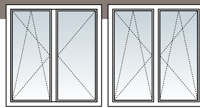
Dreh-Kipp / Dreh oder Dreh / Dreh-Kipp
