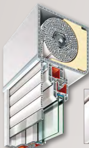
Aufsatzkasten
