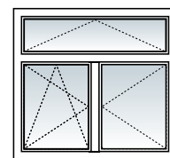
Dreh-Kipp / Dreh oder Dreh / Dreh-Kipp mit Oberlicht Kipp 1/3-2/3-Teilung Stulpausführung
