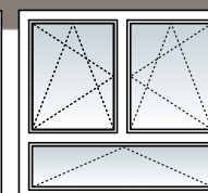
Dreh-Kipp/Dreh-Kipp mit Unterlicht Kipp 2/3-1/3-Teilung
