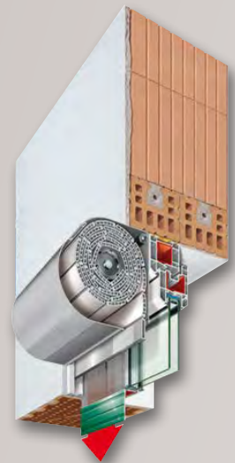
Vorbaukasten (z. B. runde Bauform mit integriertem Insektenschutz) in Fensterlaibung zurückgesetzt:
