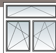
Dreh-Kipp/Dreh-Kipp mit Oberlicht Kipp 1/3-2/3-Teilung
