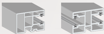
Rollladenführungsschienen – für Einfach- und Doppelführungen
