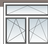
Dreh-Kipp/Dreh-Kipp mit Oberlicht Kipp 1/3-2/3-Teilung
