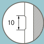
Prägung für Mala 05, 06 und 09 in Millimetern
