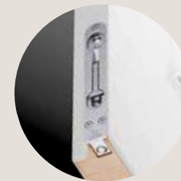
Kantenriegel unten
